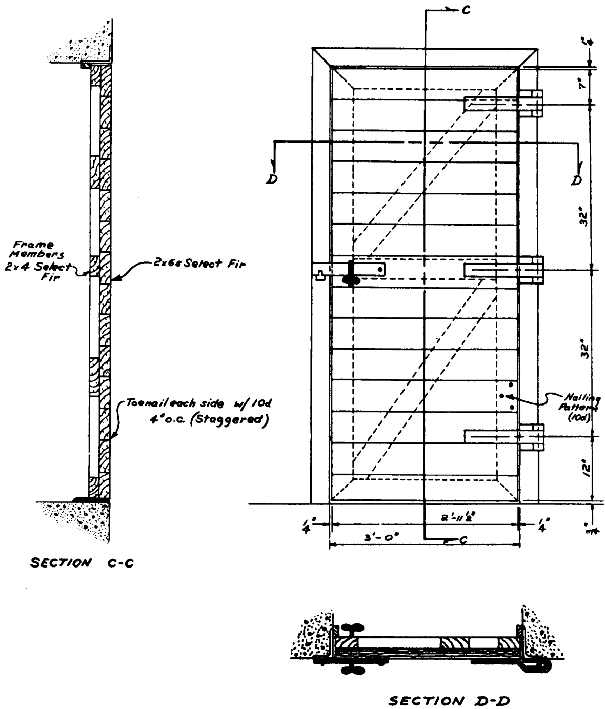
Fig. 5—Wood-plank door detail.
